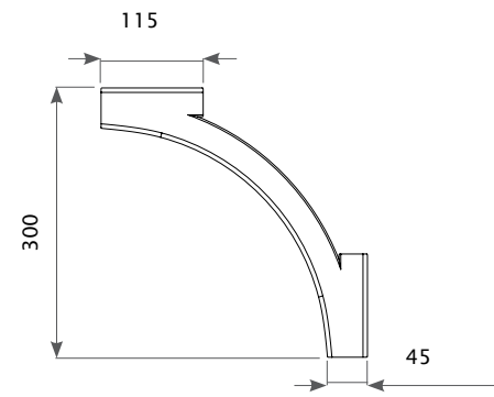
3D орнамент арт. 08 300 mm x 300 mm x 15 mm Полиуретан
