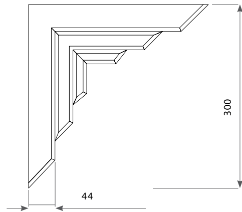
3D орнамент арт. 11 300 mm x 300 mm x 12 mm Полиуретан
