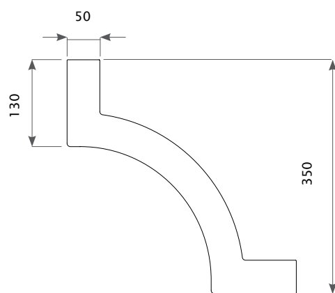
3D орнамент арт. 07 350 mm x 350 mm x 10 mm Полиуретан
