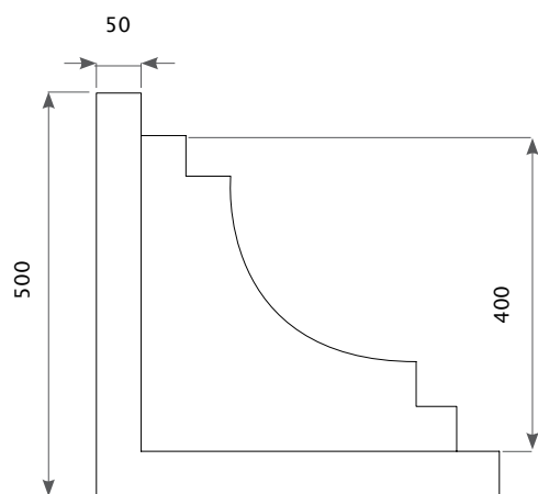
3D орнамент арт. 17 500 mm x 500 mm x 30 mm Полиуретан
