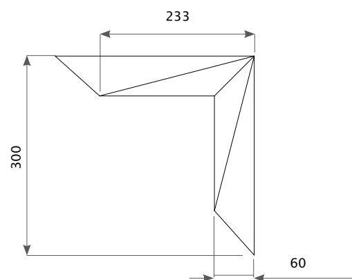
3D орнамент арт. 13 300 mm x 300 mm x 12 mm Полиуретан
