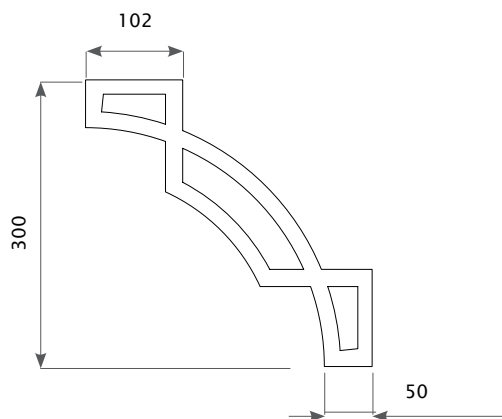
3D орнамент арт. 12 300 mm x 300 mm x 12 mm Полиуретан
